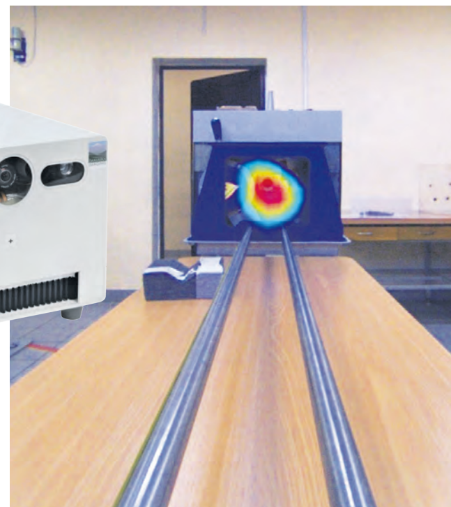
Источник радиации в поверочной установке
